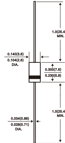
DO-15(DO-204AC)
